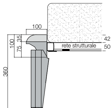
Sezione giroletto SAGOMATO CON PIEDE -P- IN LEGNO
