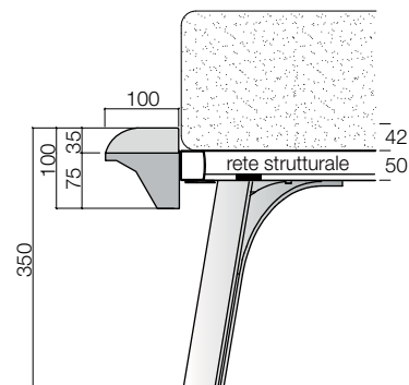
Sezione giroletto SAGOMATO CON PIEDE -V- IN METALLO SAGOMATO
