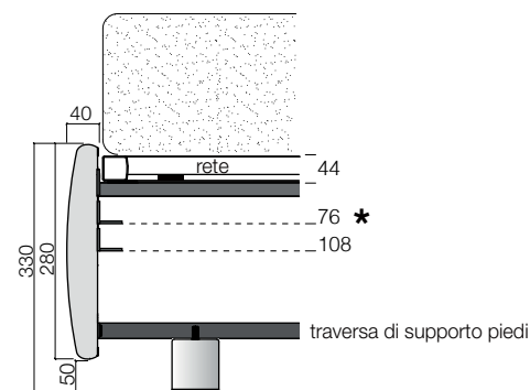
Sezione giroletto H 280 IMBOTTITO
